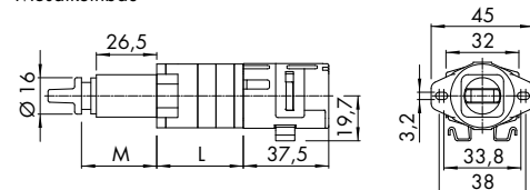
Mosaikbau
