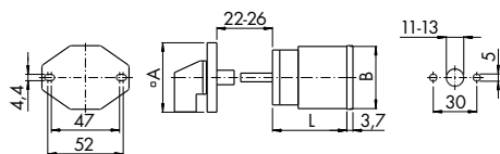
Baugröße S0
