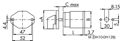
Baugröße S0
