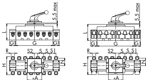
Verteilereinbau
