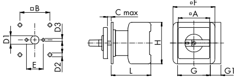
Lochbild Frontschild
