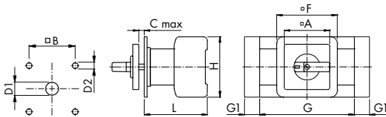
Lochbild Frontschild
