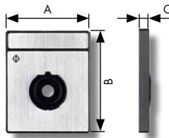
rechteckiges Frontschild
